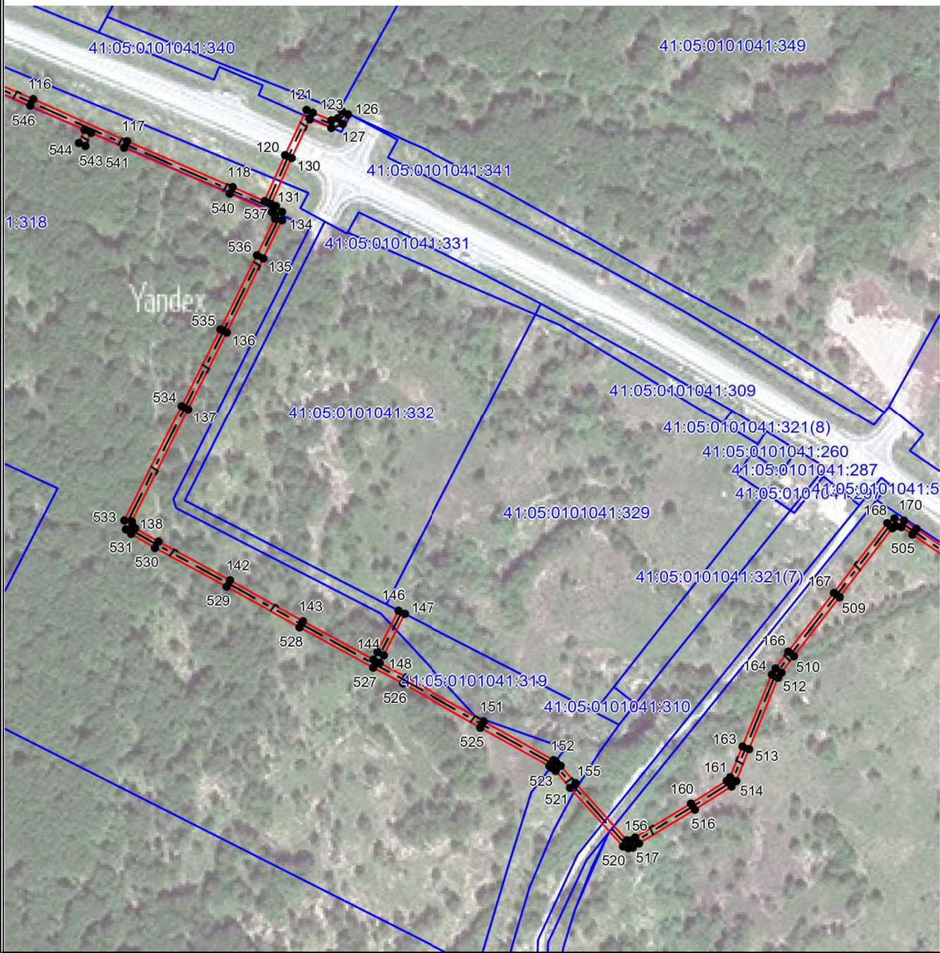
Выносной лист №9
