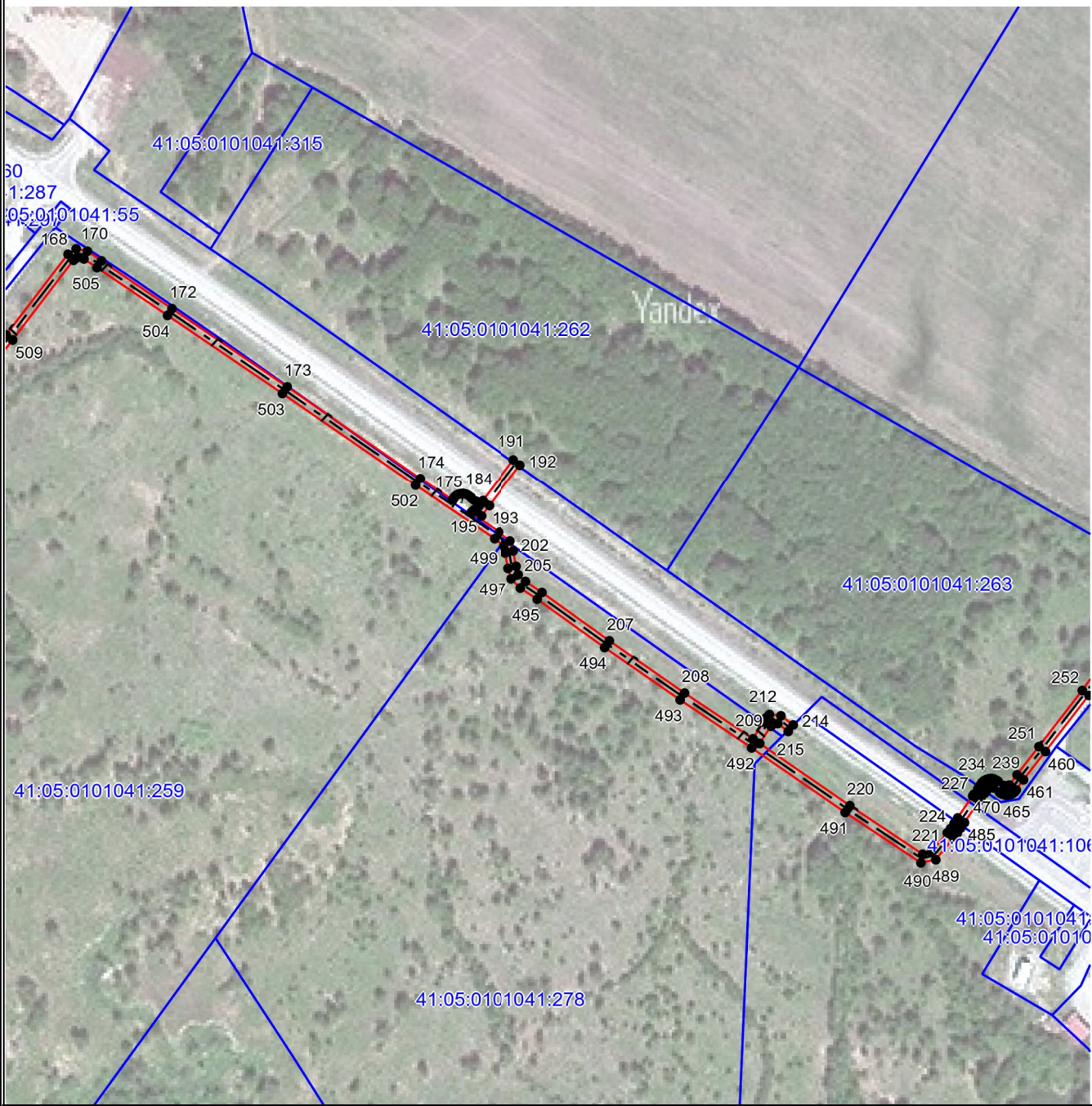
Выносной лист №10
