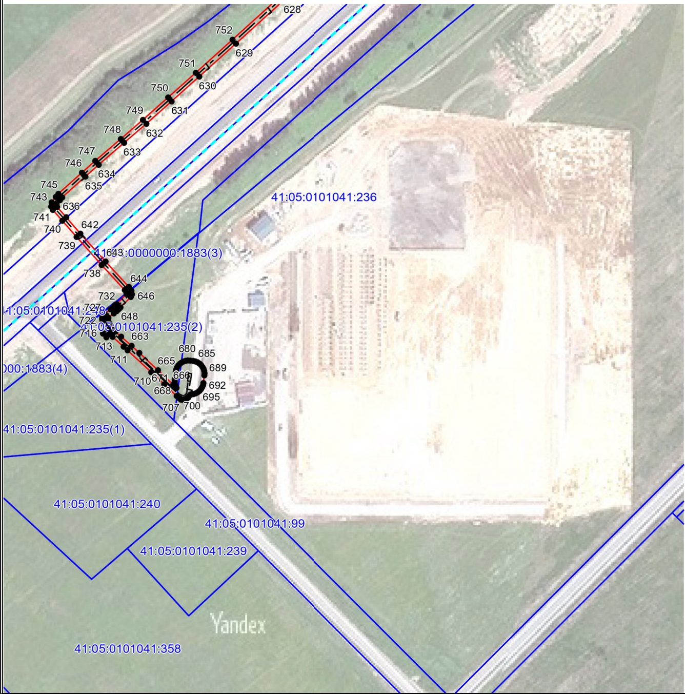
Масштаб 1:3000
