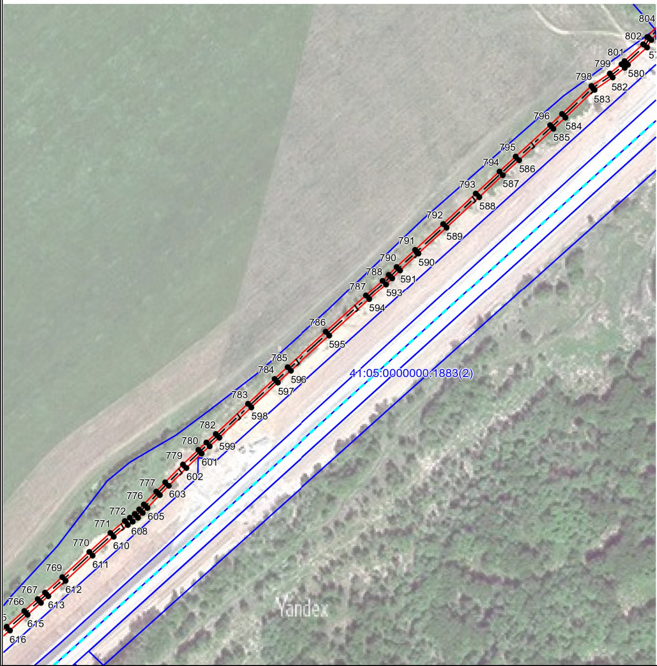
Выносной лист №3
